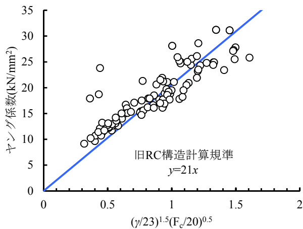
図 20 ヤング係数の新旧 RC 構造計算規準式との対応
