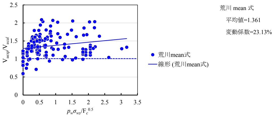
図1 荒川 mean 式の精度検定結果（一方向荷重）
