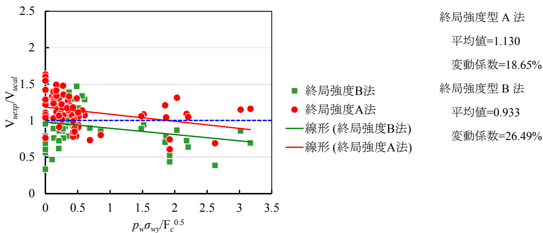
図2 終局強度型耐震設計指針式の精度検定結果（一方向荷重）
