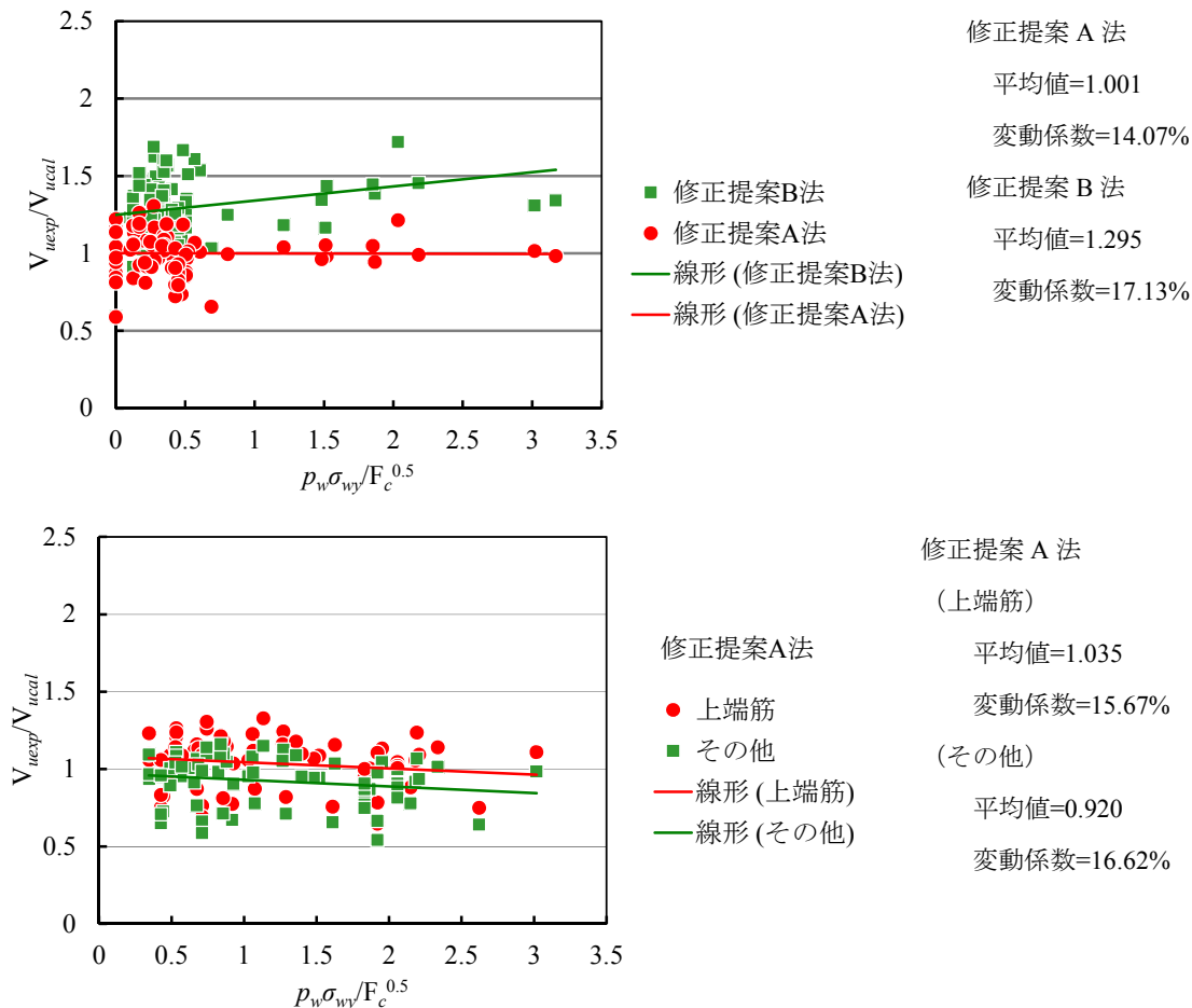
図 15 修正提案 A 法および B 法による精度検定結果
