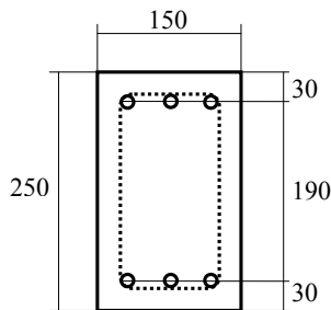
図 23 RC 梁試験体の形状寸法、配筋および荷形式
