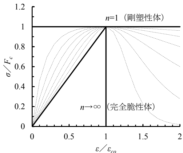
図7 Popovics 式による無次元化応力-ひずみ関係
